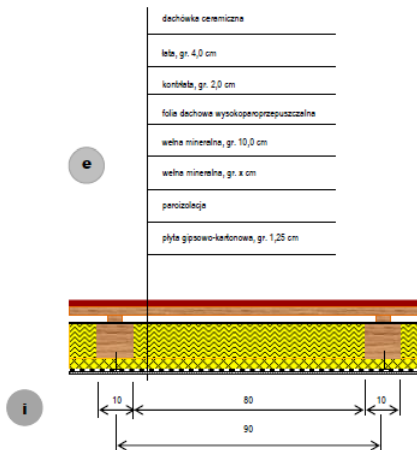
Rys. nr 06. Połączenie dachowe docieplone.
